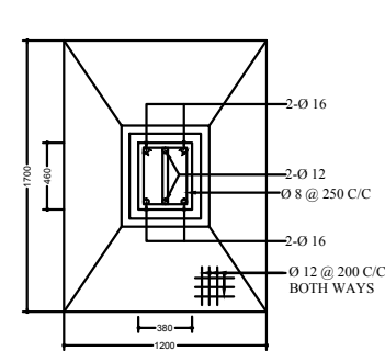
PLAN COLUMN -C 5
