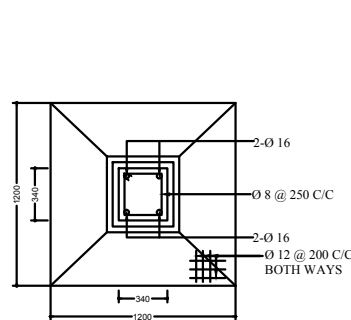
PLAN COLUMN -C 4
