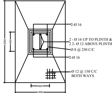
PLAN COLUMN -C 3
